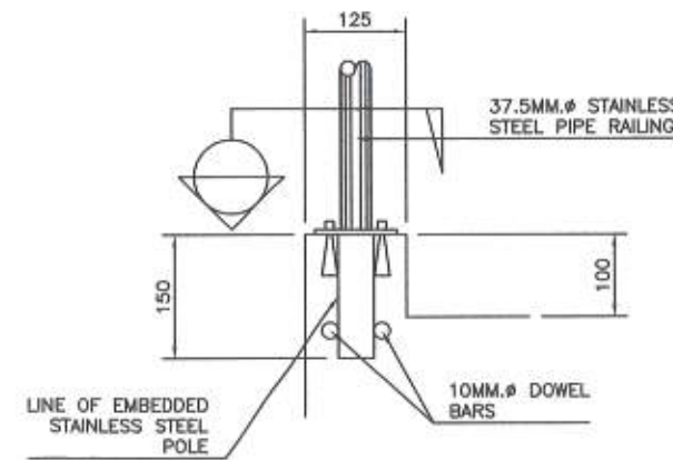
DETAIL SCALE 1:5 M.
