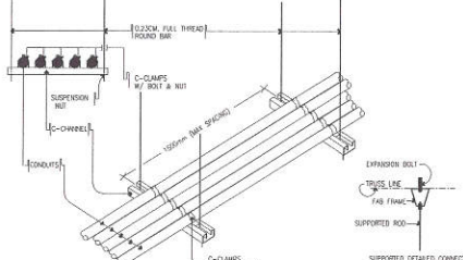
TRAPEZE TYPE CONDUIT ARRANGEMENT
