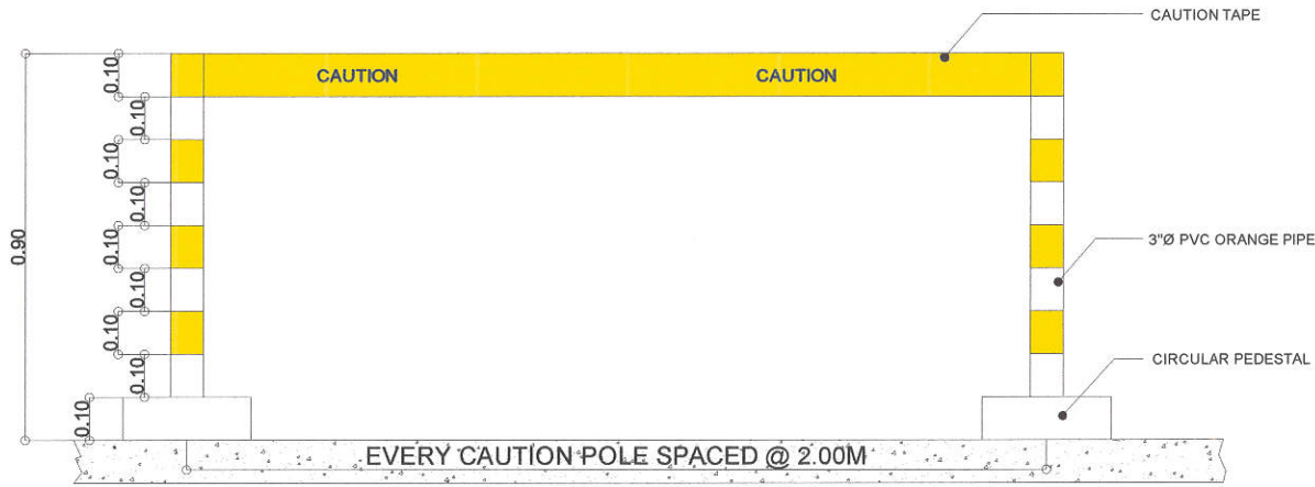
ELEVATION
