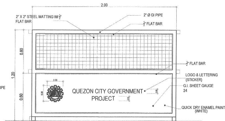
ELEVATION
