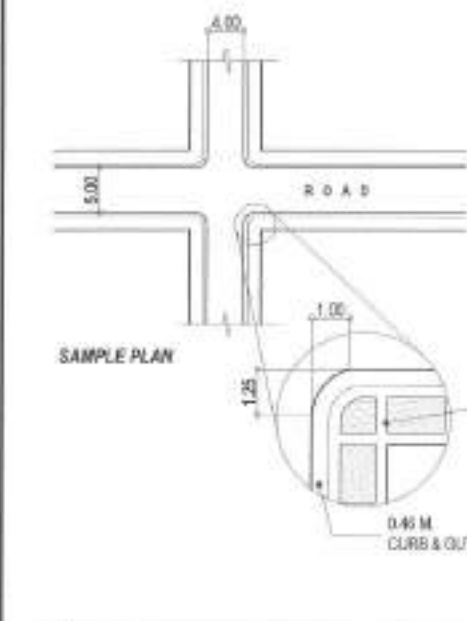
3 CHAFPLAN DETAIL SCALE : NTS
