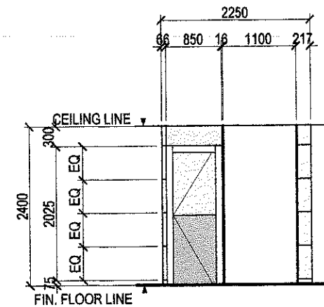
ELEVATION "C"
