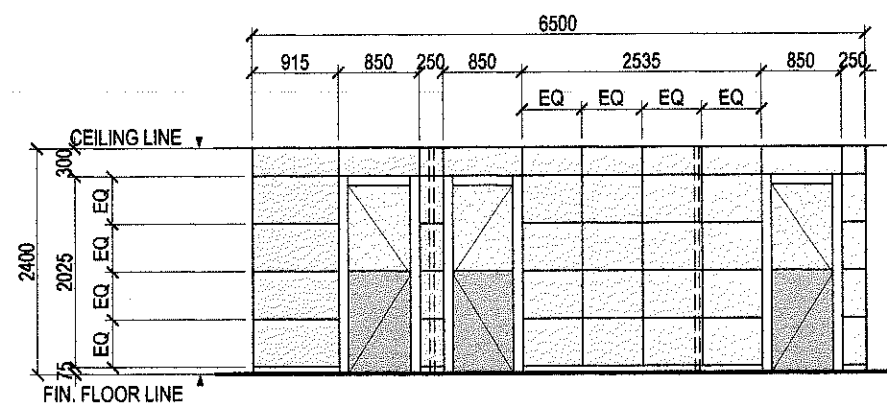
ELEVATION 'C'
