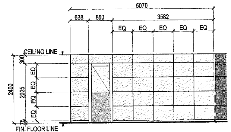
ELEVATION 'E'
