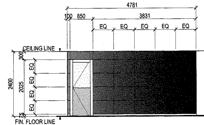
ELEVATION 'B'
