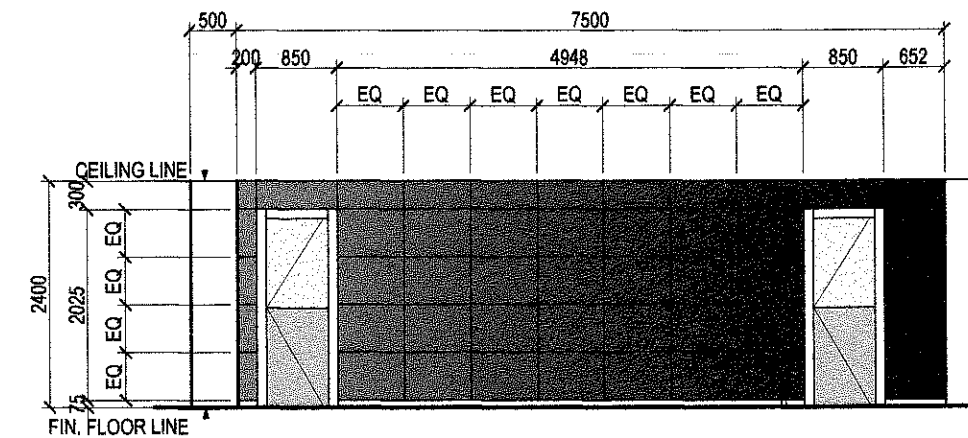
ELEVATION 'B'
