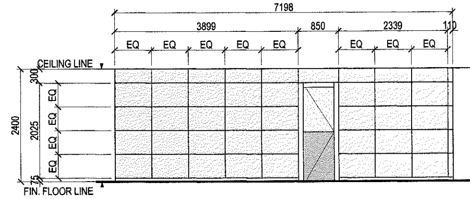
ELEVATION 'C'
