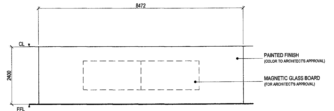
ELEVATION 'C' / 'D'
