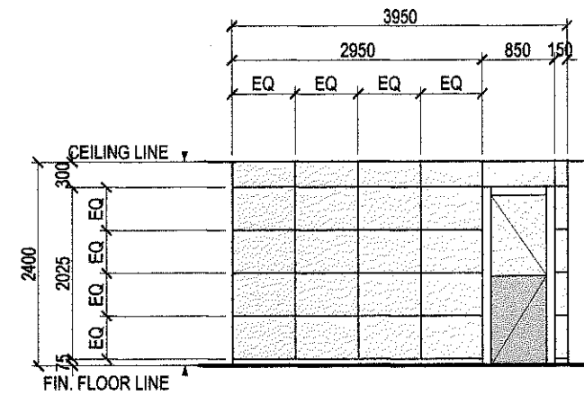
ELEVATION 'C' / 'D'
