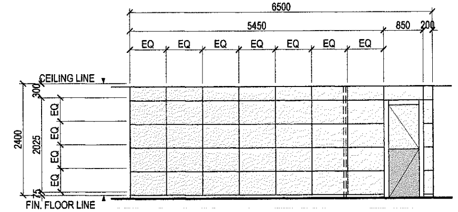
ELEVATION 'E'
