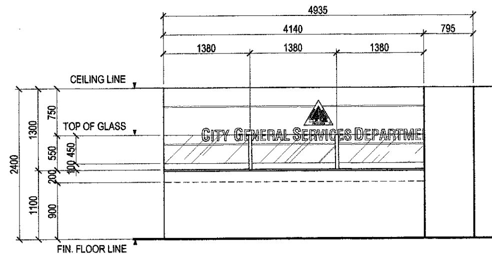
ELEVATION 'B'
