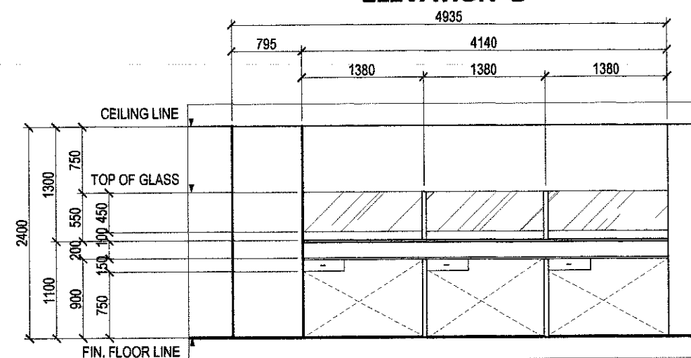
ELEVATION 'B'
