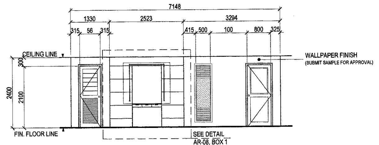
ELEVATION 'E'
