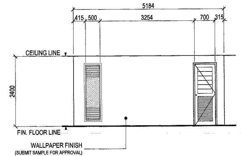
ELEVATION "C"
