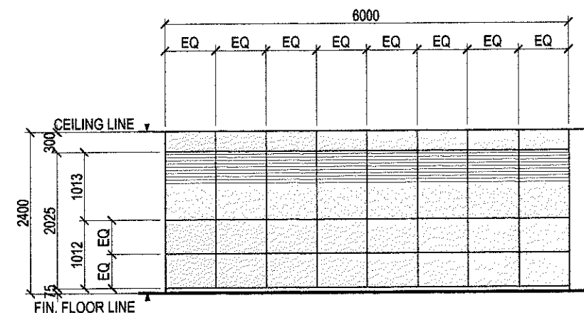
ELEVATION 'G'
