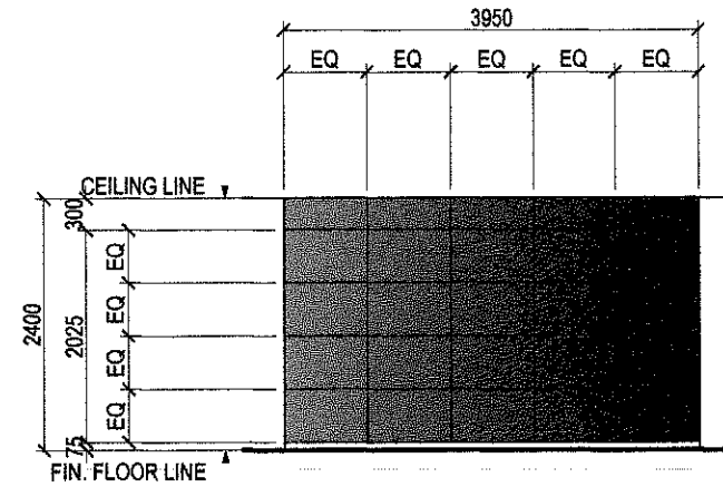
ELEVATION 'B'
