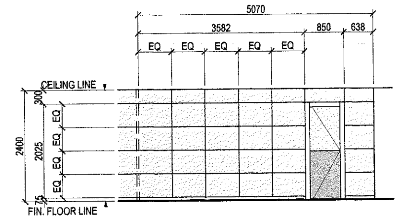
ELEVATION 'F'
