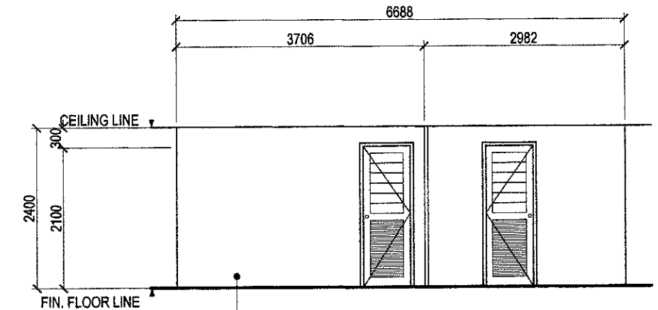
ELEVATION 'F'
