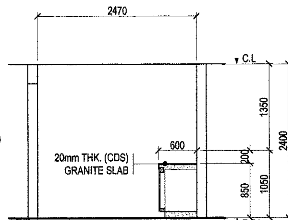
SECTION THRU 'B'
