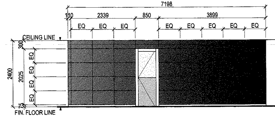
ELEVATION 'D'
