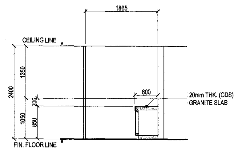
SECTION THRU 'B'
