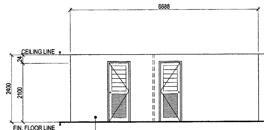
ELEVATION 'E'
