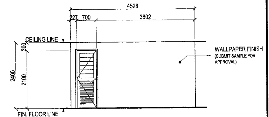
ELEVATION 'D'
