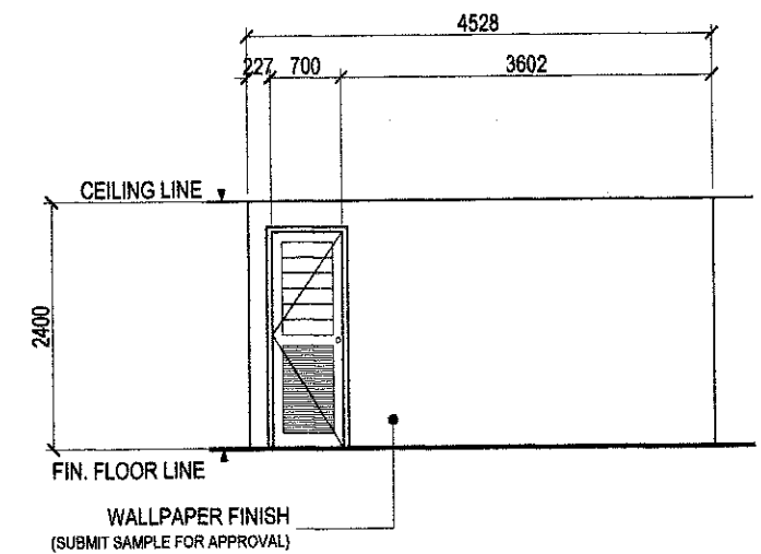
ELEVATION 'D'
