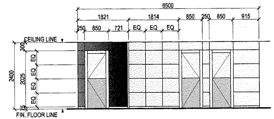
ELEVATION 'D'
