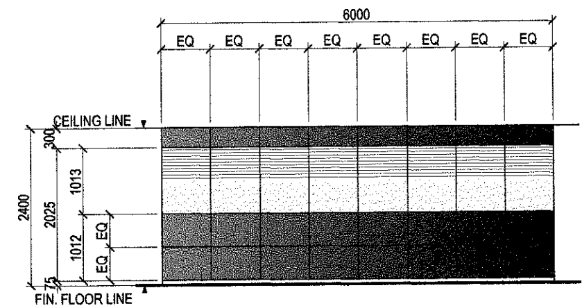
ELEVATION 'H'
