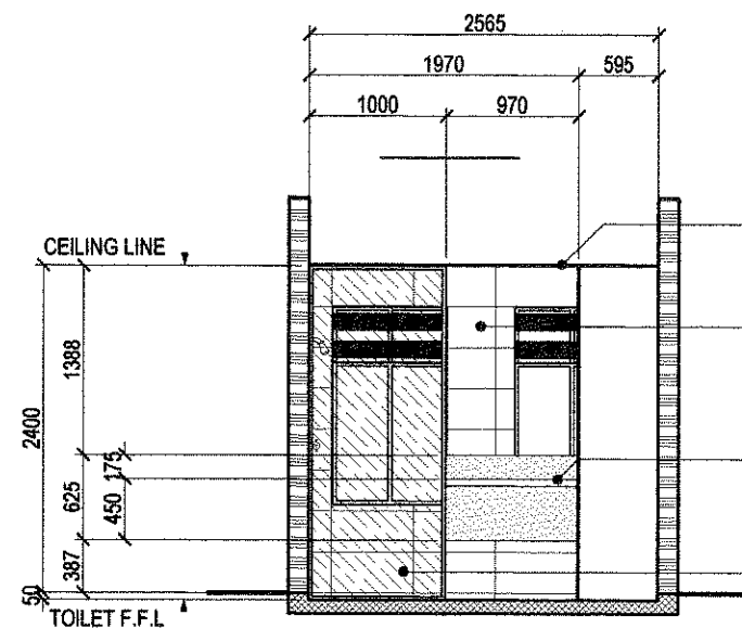
SECTION THRU 'B'
