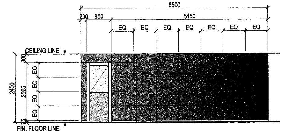
ELEVATION 'F'
