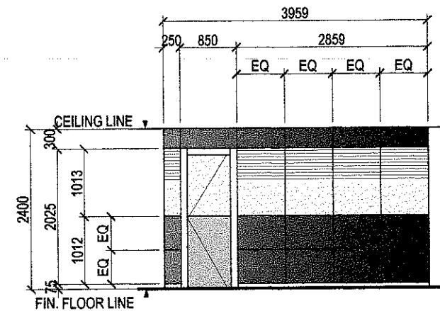
ELEVATION 'D'
