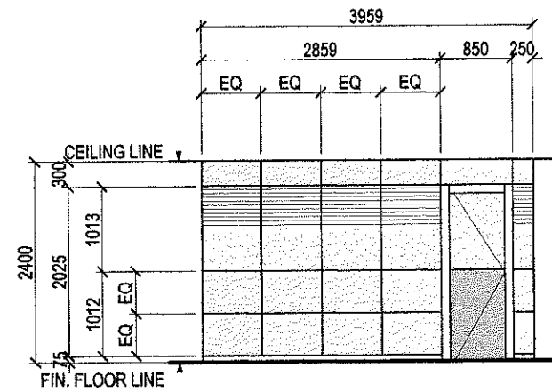
ELEVATION 'C'
