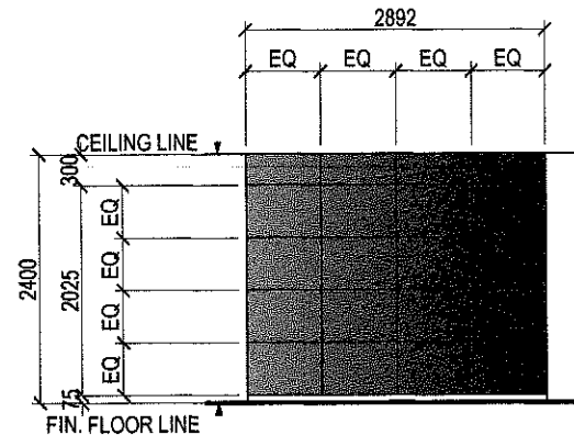
ELEVATION 'B'
