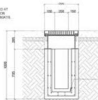
ELEVATION SECTION SCALE: 1:20MTS
