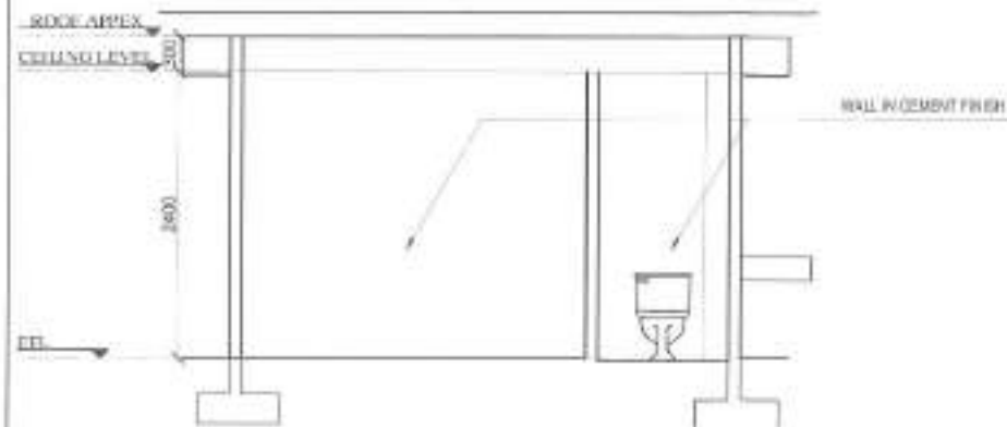
4 SECTION-1 A3 SCALE 1:50
