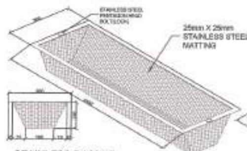
STAINLESS BASKET SCALE: 1:10MTS
