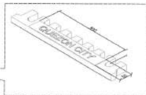
STAINLESS BASKET SCALE: 1:10MTS
