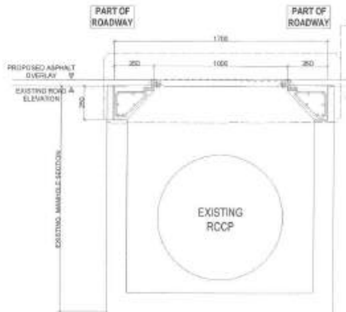
SECTION SCALE: 1:200
