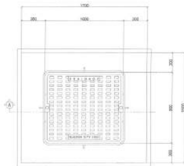
PLAN SCALE: 1:200
