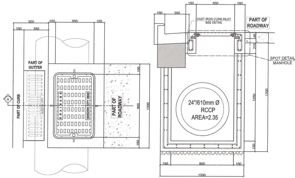
PLAN SCALE: 1:20MTS
