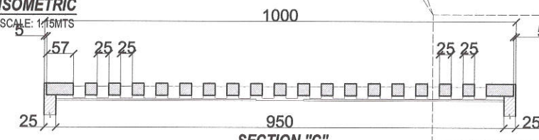
SECTION "C" SCALE: 1:8MTS
