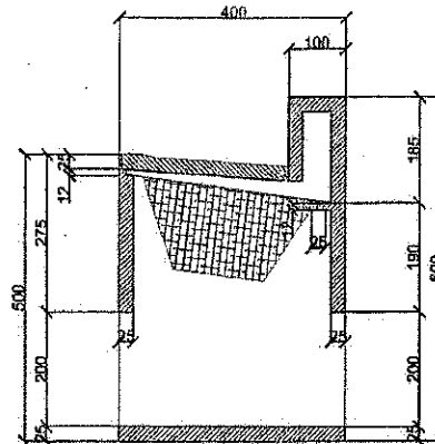
SECTION "A" SCALE: 1:10MTS
