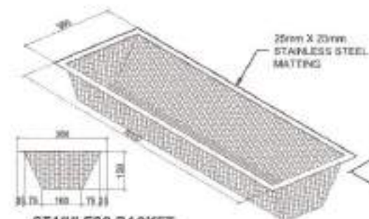
STAINLESS BASKET SCALE: 1:10MTS
