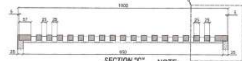
SECTION "C" SCALE: 1:10MTS
