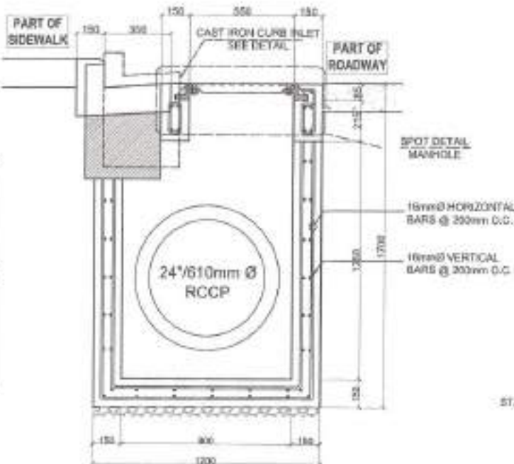
ELEVATION SECTION SCALE: 1:20MTS
