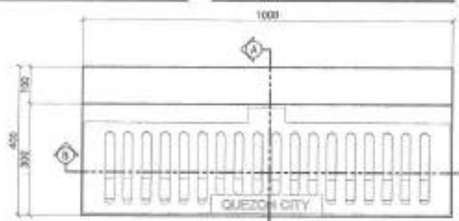
TOP VIEW SCALE: 1:10MTS
