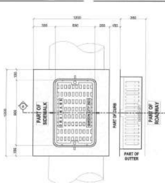
PLAN SCALE: 1:20MTS
