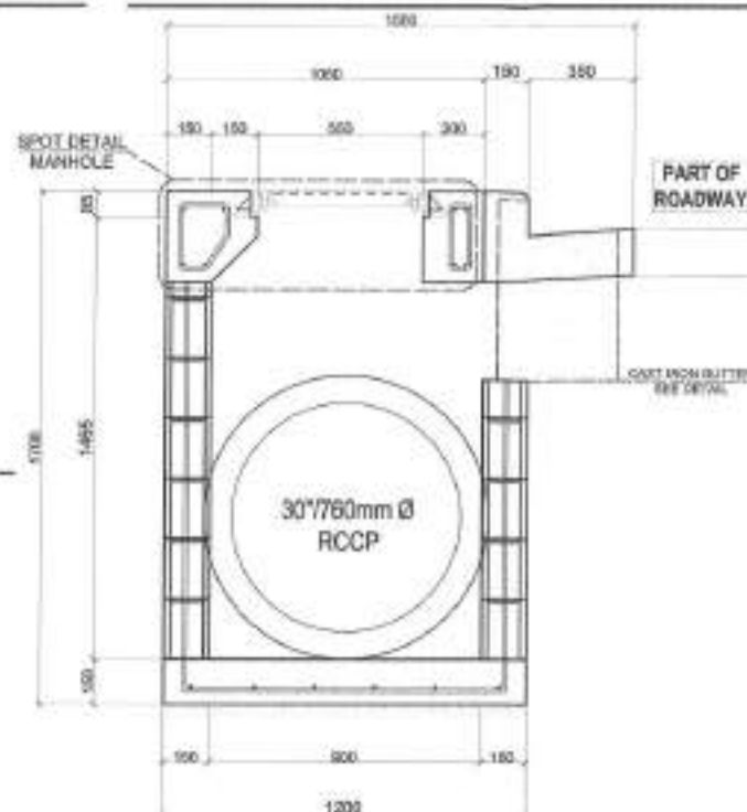
ELEVATION SECTION SCALE: 1:20MTS
