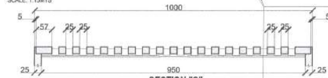
SECTION "C" SCALE: 1:8MTS
