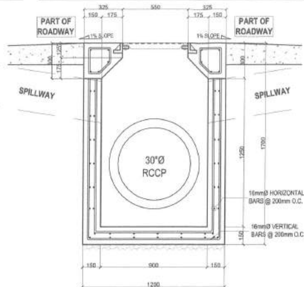
ELEVATION SECTION SCALE: 1:20MTS
