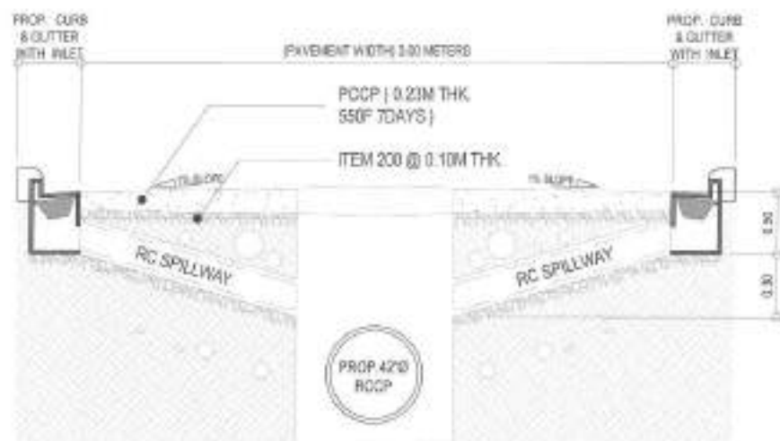
1 ROADWAY SECTION A (STA. 00+000 TO STA. 00+026)
