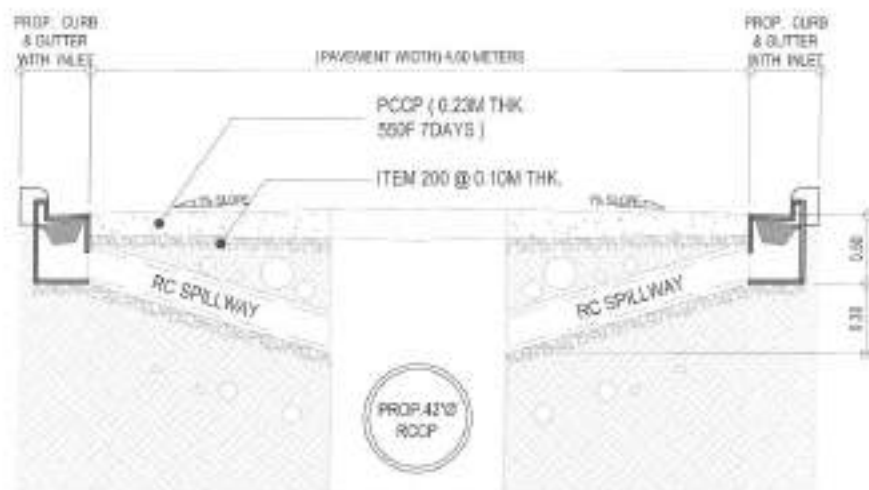
1 ROADWAY SECTION C(STA. 00+068 TO STA. 00+128)
