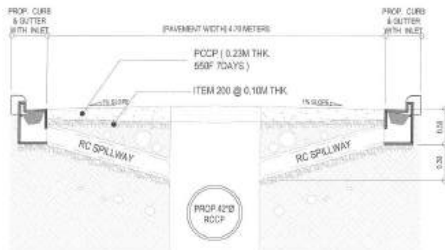
3 ROADWAY SECTION B(STA. 00+026 TO STA. 00+068)
