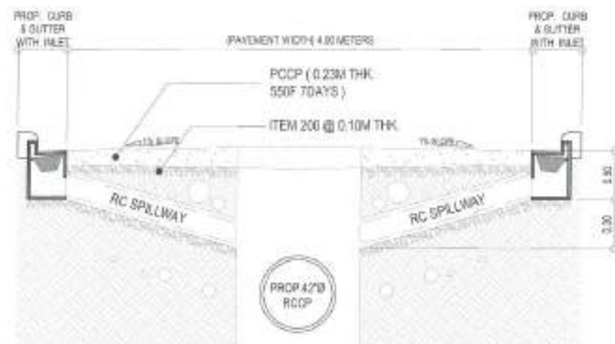
2 ROADWAY SECTION D(STA. 00+136 TO STA. 00+322)
