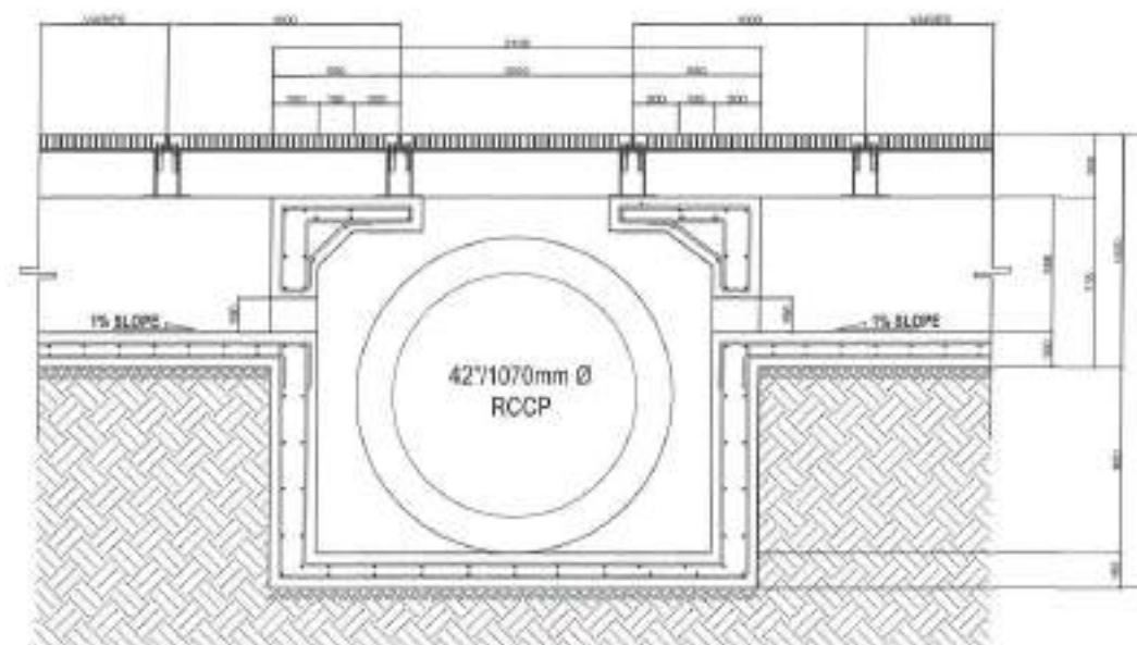
ELEVATION SECTION SCALE: 1:30MTS
