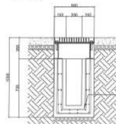
ELEVATION SECTION SCALE: 1:30MTS
