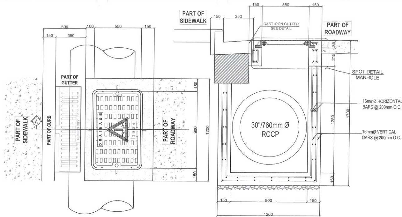
PLAN SCALE: 1:20MTS
