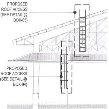
2 ELEVATION "A"
